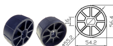
Polea 60 redondo | 61.005.012
